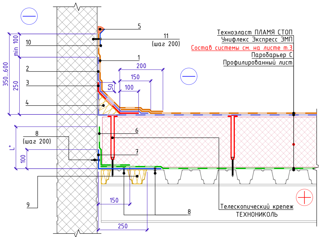
Спецификация на узел У.3.1-2020.09
