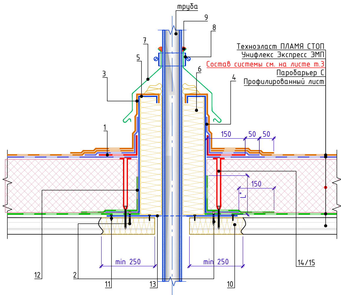
Спецификация на узел У.7.3-2020.09
